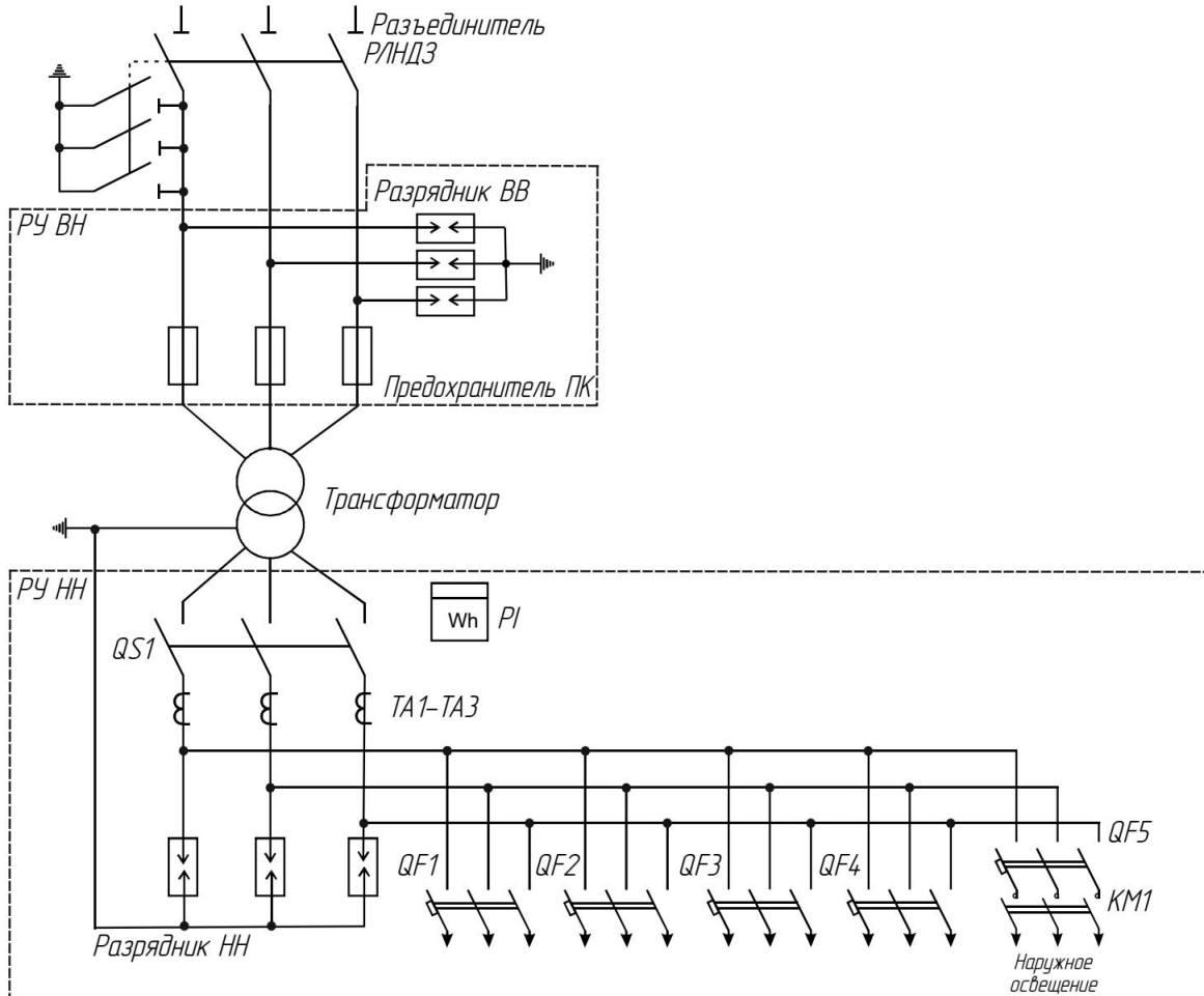
Однолинейная схема СТП
